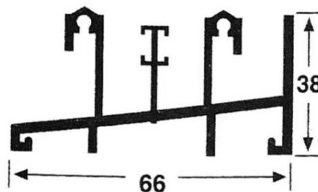
2514 RIEL INFERIOR 4 PATAS Peso: 1.013 Kg/M Espesor: 1.3 mm
