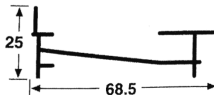
2015 ZOCALO ALTO Peso: 0.613 Kg/M Espesor: 1.3 mm
