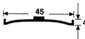
4506 TALONERA Peso: 0.189 Kg/M Espesor: 1.3 mm
