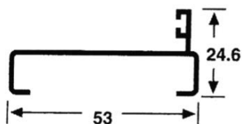
4503 MARCO PUERTA Peso: 0.356 Kg/M Espesor: 1.3 mm
