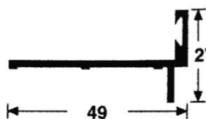
4508 TRASLAPO Peso: 0.354 Kg/M Espesor: 1.5 mm
