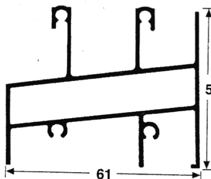
2013 RIEL C/CAMARA DE AGUA Peso: 1.115 Kg/M Espesor: 1.3 mm
