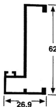
4502 MARCO PUERTA Peso: 0.507 Kg/M Espesor: 1.4 mm
