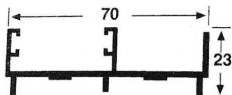
2509 JAMBA Peso: 0.556 Kg/M Espesor: 1.3 mm
