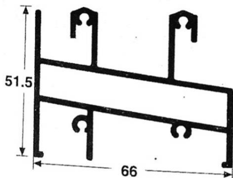
2513 RIEL C/CAMARA DE AGUA Peso: 1.164 Kg/M Espesor: 1.3 mm
