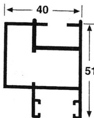
2512 BATIENTE REFORZADO Peso: 0.843 Kg/M Espesor: 1.5 mm
