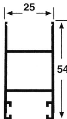
2517 BATIENTE TERMOPANEL Peso: 0.576 Kg/M Espesor: 1.3 mm
