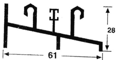
2014 RIEL ZONAS LLUVIOSAS Peso: 0.662 Kg/M Espesor: 1.3 mm
