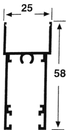
2516 ZOCALO REFORZADO TERMOPANEL Peso: 0.642 Kg/M Espesor: 1.3 mm
