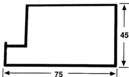
4501 BASTIDOR Peso: 0.508 Kg/M Espesor: 1.4 mm
