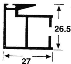
2011 TRASPASO REFORZADO Peso: 0.460 Kg/M Espesor: 1.3 mm
