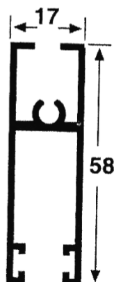
2015 ZOCALO ALTO Peso: 0.613 Kg/M Espesor: 1.3 mm
