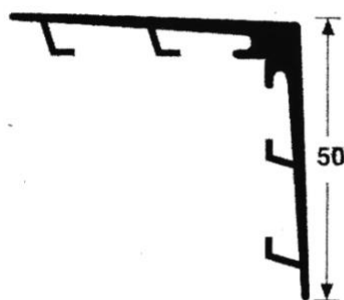
4213 ESCUADRA Peso: 0.968 Kg/M Espesor: 1.5 mm
