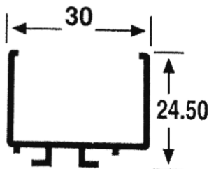
2520 ADAPTADOR TERMOPANEL Peso: 0.300 Kg/M Espesor: 1.3 mm
