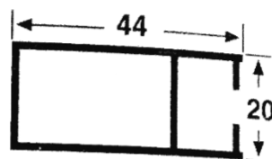
2010 BATIENTE Peso: 0.467 Kg/M Espesor: 1.3 mm
