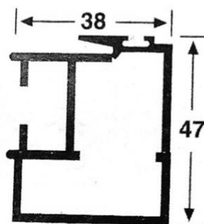
2511 TRASLAPO REFORZADO Peso: 0.806 Kg/M Espesor: 1.5 mm
