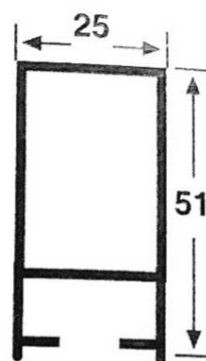
2510 BATIENTE Peso: 0.559 Kg/M Espesor: 1.3 mm
