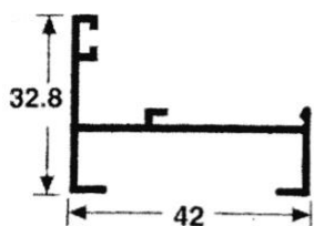
4209 MARCO Peso: 0.415 Kg/M Espesor: 1.4 mm
