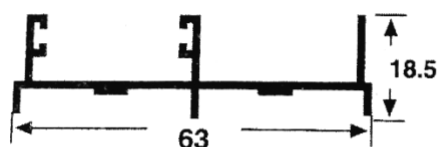
2009 JAMBA Peso: 0.448 Kg/M Espesor: 1.3 mm
