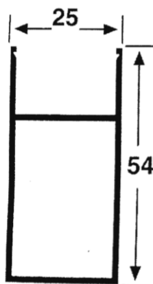
2518 BATIENTE TERMOPANEL Peso: 0.538 Kg/M Espesor: 1.3 mm
