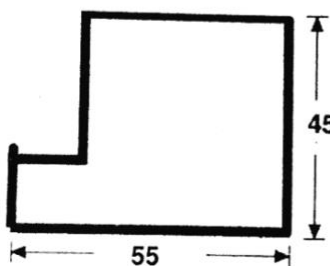
4507 BASTIDOR Peso: 1.040 Kg/M Espesor: 2.0 mm
