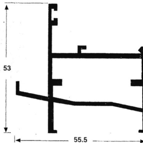
4219 MARCO CAMARA DE AGUA Peso: 0.738 Kg/M Espesor: 1.4 mm
