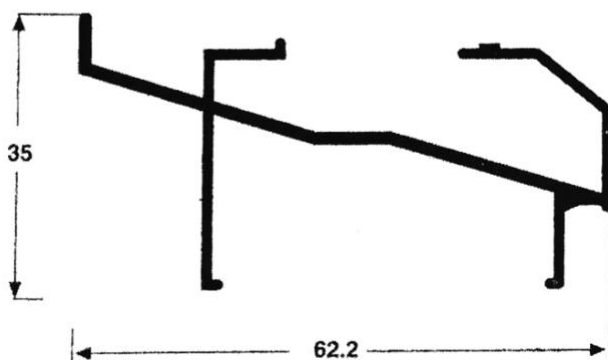
4210-A CAMARA DE AGUA LINEA 42 NUEVO Peso: 0.600 Kg/M Espesor: 1.4 mm
