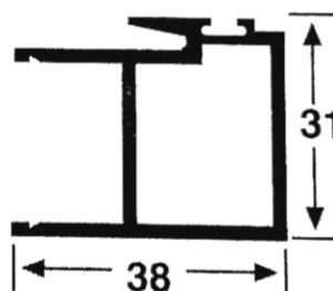
2519 TRASLASO TERMOPANEL Peso: 0.521 Kg/M Espesor: 1.3 mm
